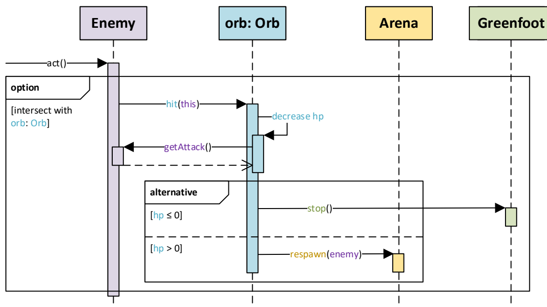
Obrázek 7: UML sekvenční diagram interakce instance třídy Enemy s jinými objekty při dosáhnutí instance třídy Orb
